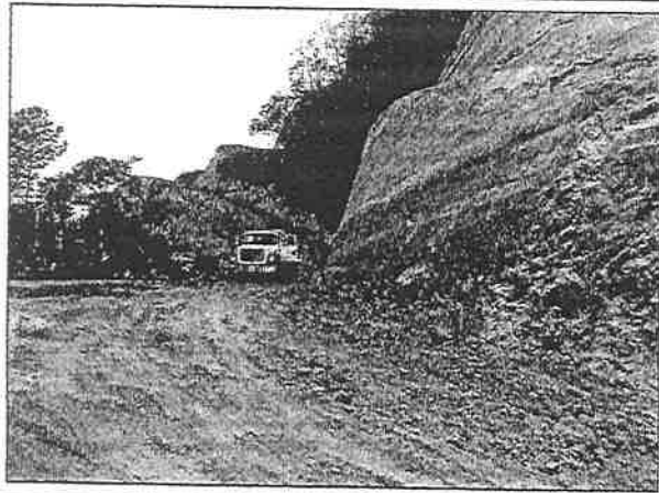
Corte de material rocoso en Est. 269.820.00 L.D.
